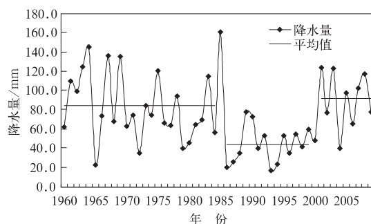
图 1 1960—2009 年陕西北部 9 月降水量变化曲线
