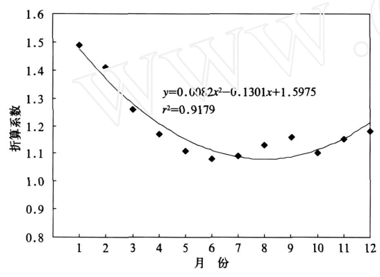
图 5 比对系数月平均值的变化曲线
