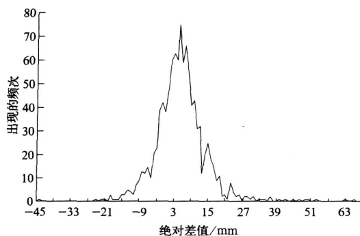
图 1 月蒸发量绝对差值的频率分布图
