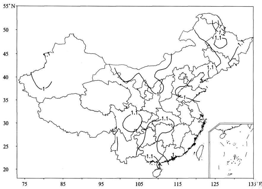
图 4 我国蒸发量观测期间比对系数等值线分布图
