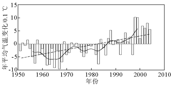
图 1 1951—2004 年青藏高原年平均气温距平变化
