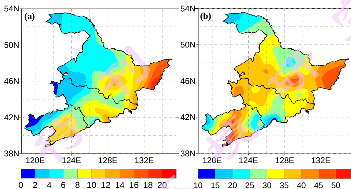
图 3 东北地区冬季降雪量绝对误差(mm)和相对误差(%)的空间分布
