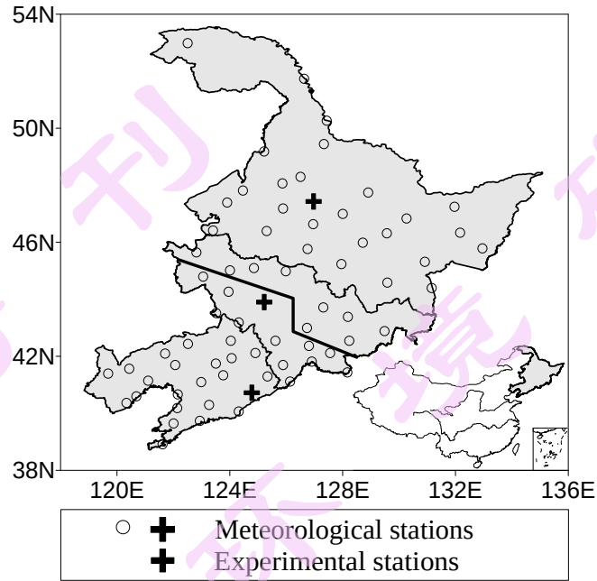
图 1 研究区域、对比试验站点和气象站点分布以及分区
