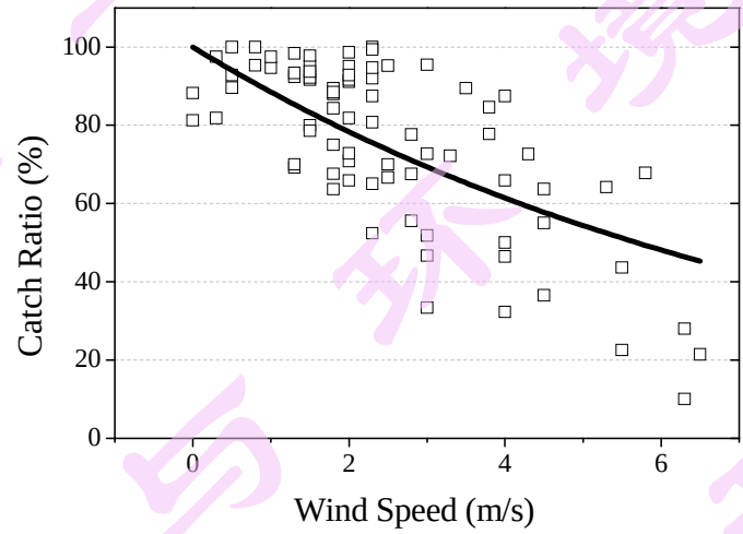
图 2 日平均风速与普通雨量计捕获率之间的关系（降雪量大于 1.0mm）
