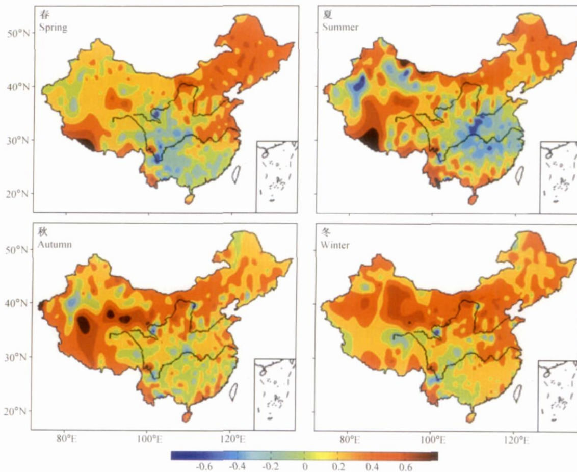
图4 1951~2004年中国大陆季节平均气温的趋势
